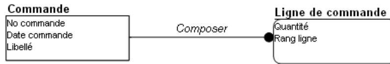
Relation obligatoire identifiante
