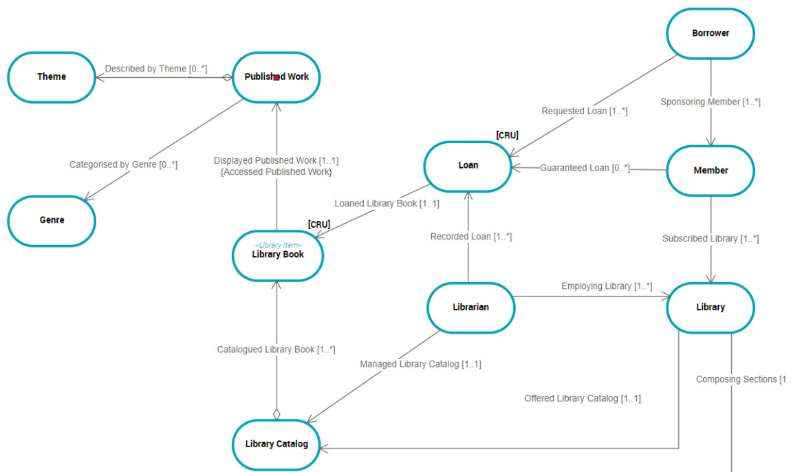
Diagramme de concept avec les vues standards
